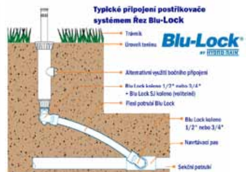
Typické připojení postřikovače systémem Řez Blu-Lock Blu Lock® strana 23
