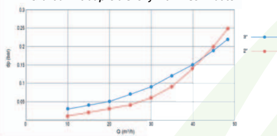
Graf tlak. ztrát pro diskový filtr 2" semi-auto
