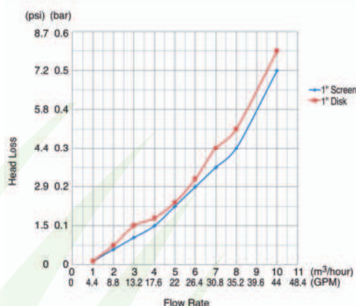
Graf tlakových ztrát pro filtr 1"
