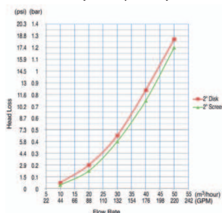
Graf tlakových ztrát pro síťový filtr 2"
