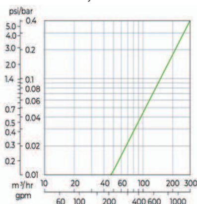
Tlakové ztráty SIGMA PRO 6" a 8"
