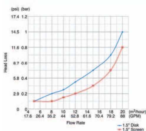
Graf tlakových ztrát pro filtr 6/4"
