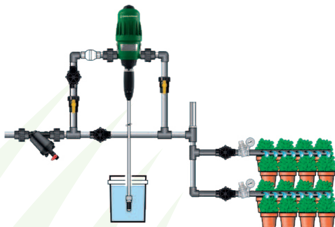
vzorové schéma instalace dávkovacího čerpadla
