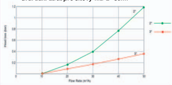
Graf tlak. ztrát pro síťový filtr 2" semi-
