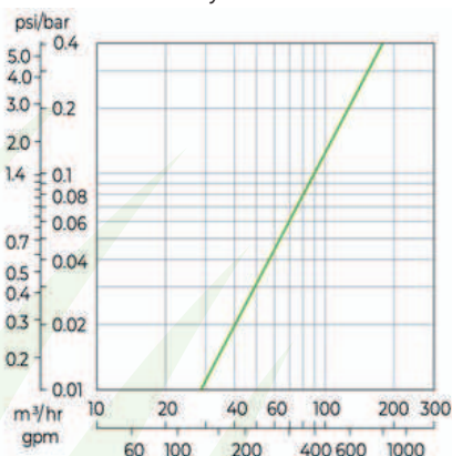
Tlakové ztráty SIGMA PRO 4'
