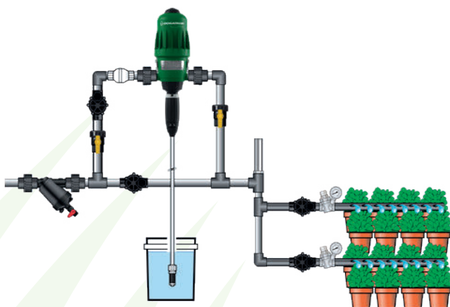
vzorové schéma instalace dávkovacího čerpadla
